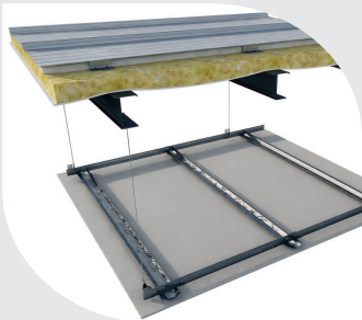
Cubiertas metálicas
